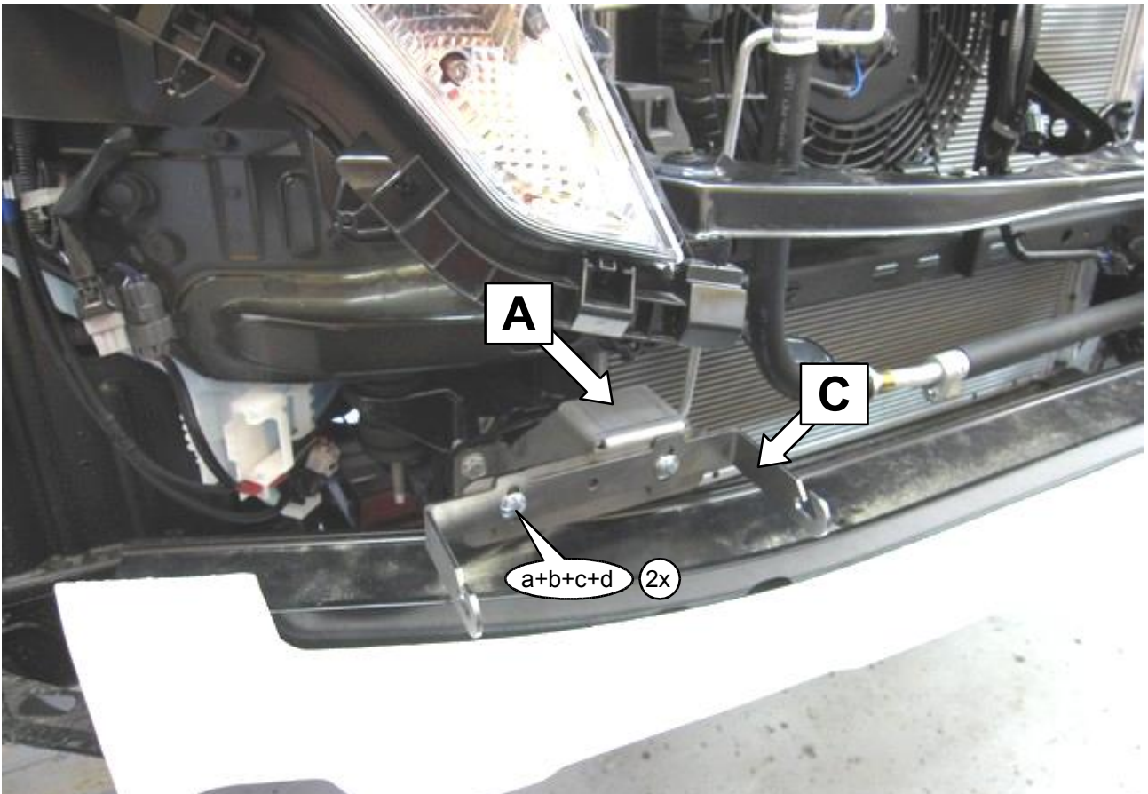
5 Rechte Seite / Right side
