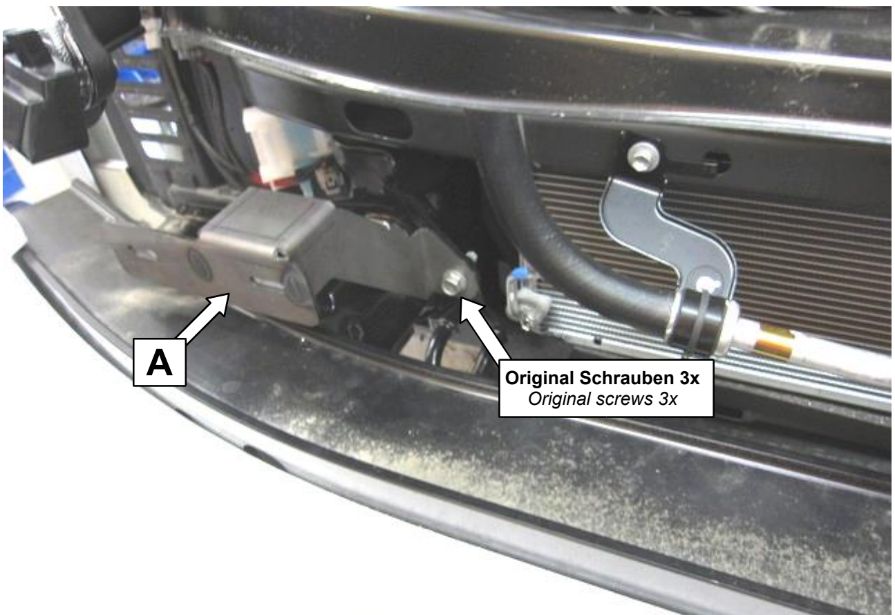
4 Rechte Seite, das gleiche auf der linken Seite! Right side, the same on the left side! This caption block contains the number '4' in a box on the left and the text 'Rechte Seite, das gleiche auf der linken Seite!' and 'Right side, the same on the left side!' in a larger box on the right.
